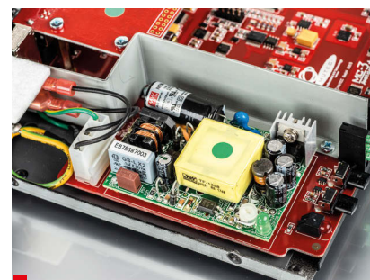
Zasilacz MC3+ bazuje na module Meanwell.
