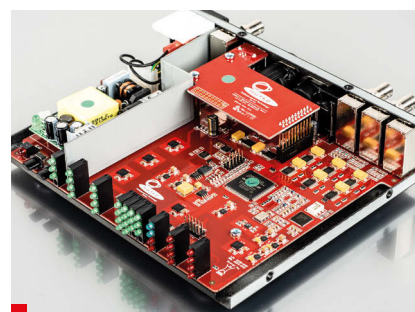
Wewnątrz MC3+ zwraca uwagę procesor FPGA Altera Cyclone III i opatentowane moduły złącz BNC.
